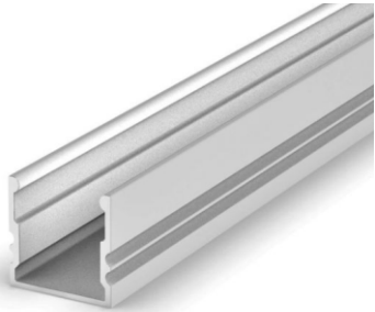
PROFIL OŚWIETLENIOWY LED PROSTY SREBRNY ANODOWANY 1,5x200 cm
